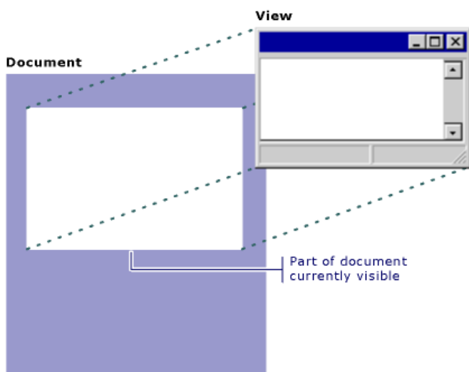
Slika 6 Prikaz dokument/pogled veze
